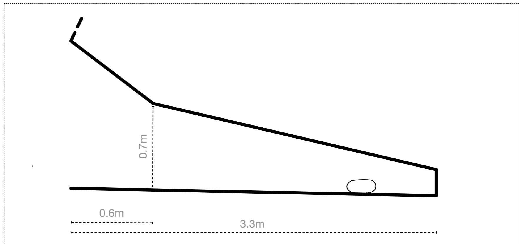
Sivuleikkaus A-A
