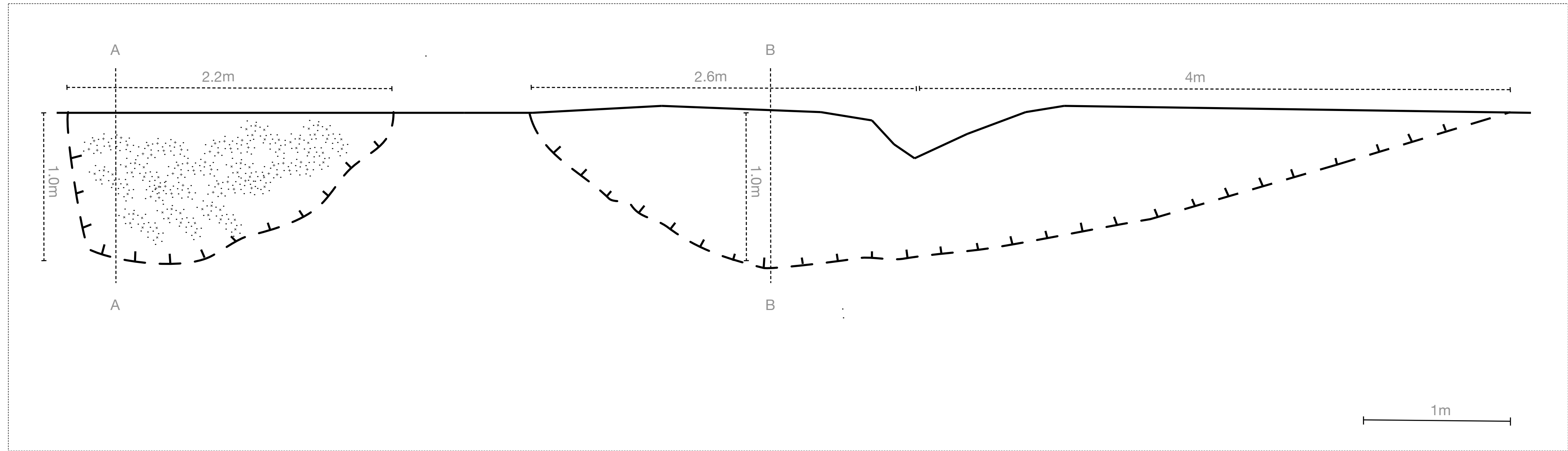
Sivuleikkaus A-A
