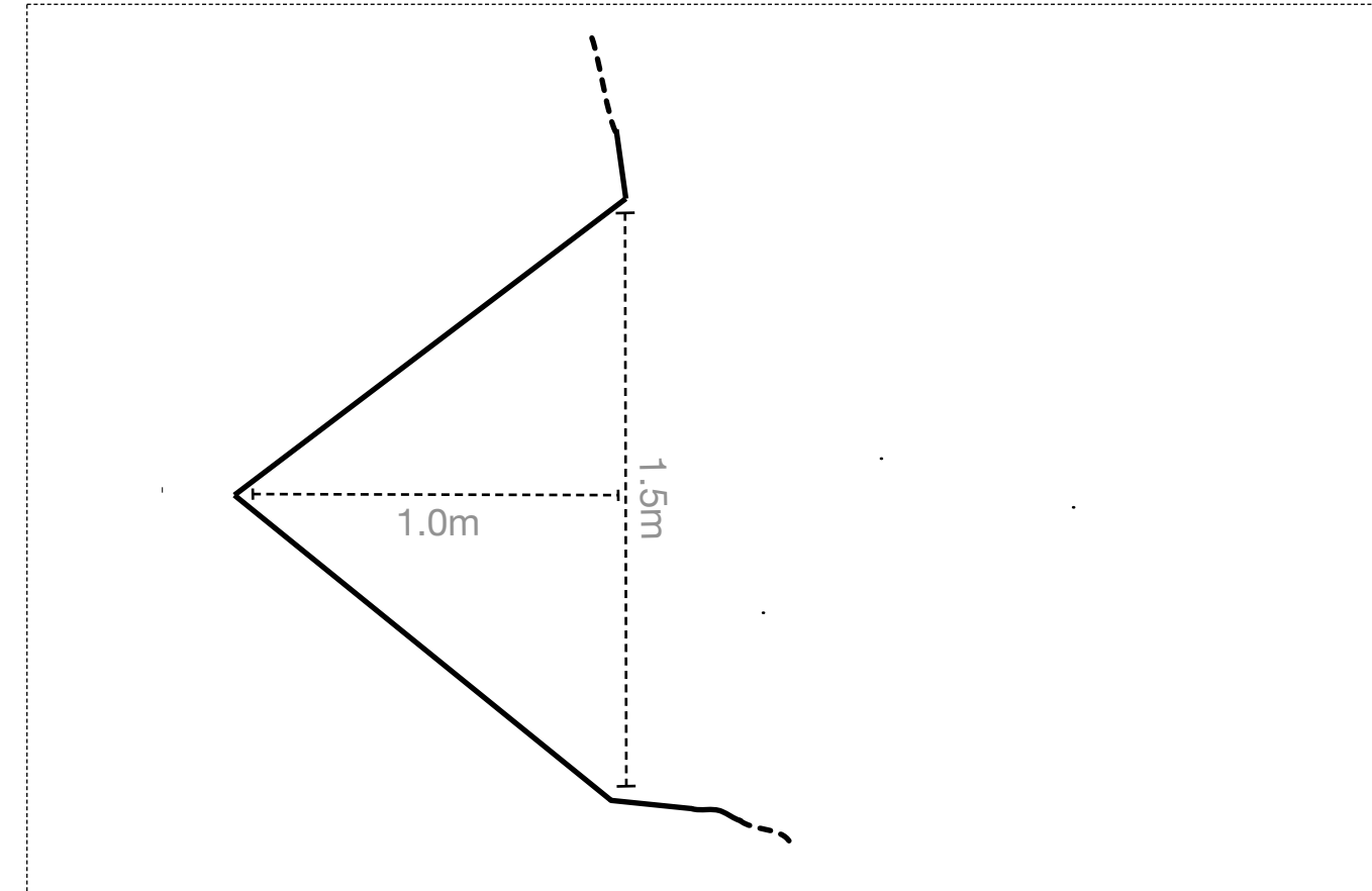
Sivuleikkaus B-B
